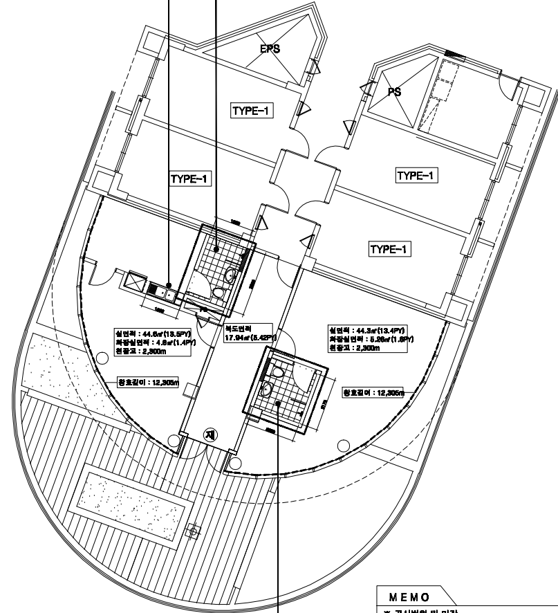
기존도어 철거 후 1.0B조적쌓기 확장실 구획 신설 (도어신설)
